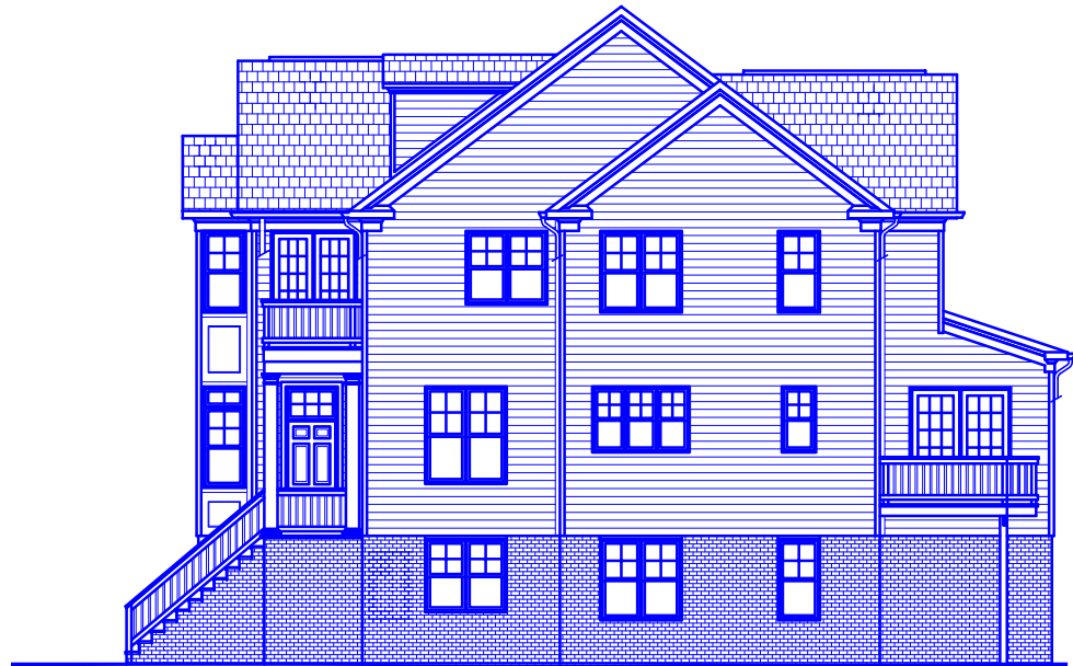
RIGHT ELEVATION
